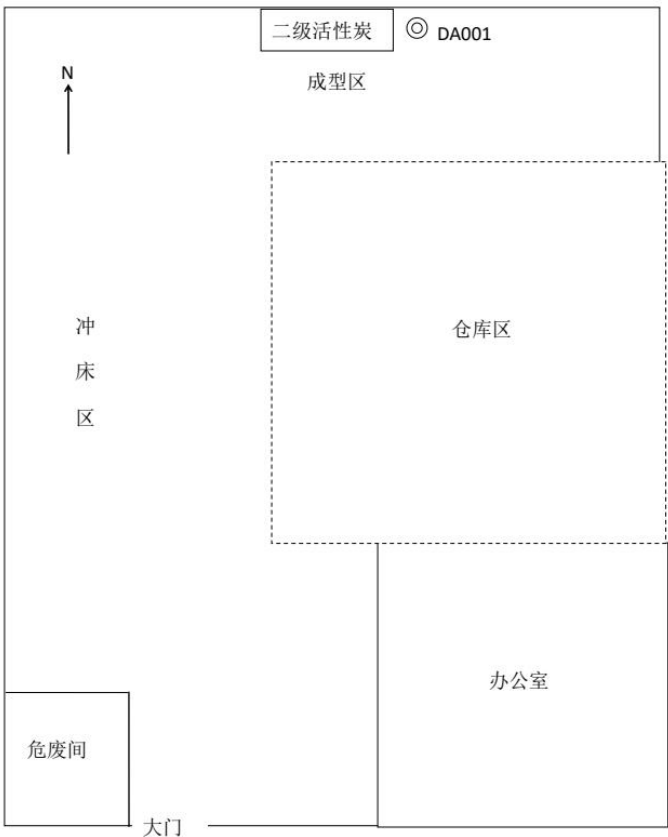
图 2-3 厂区平面布置图
